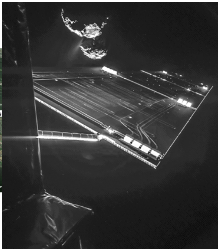
Изображение: ESA/Rosetta/Philae/CIVA
