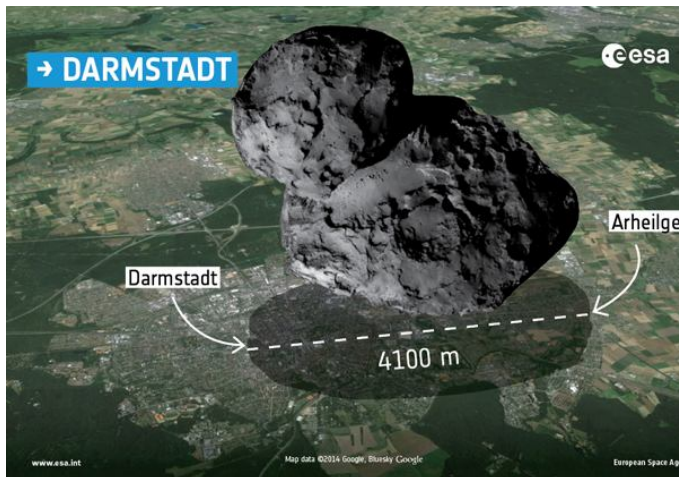
Изображение: ESA/Rosetta/Navcam
