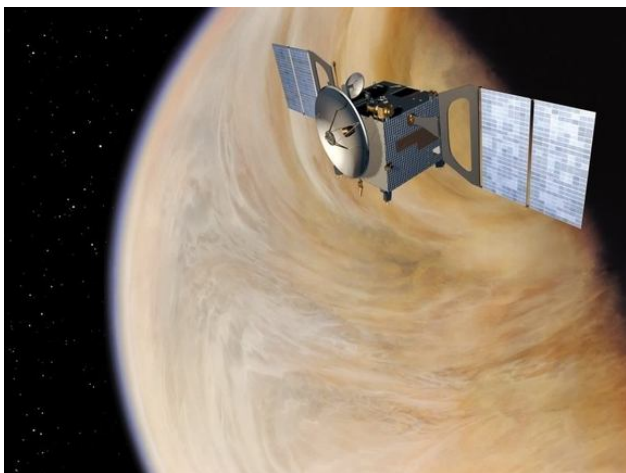
Venus Express у Венеры.
