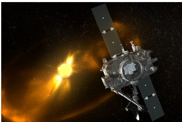
Один из аппаратов Stereo.
